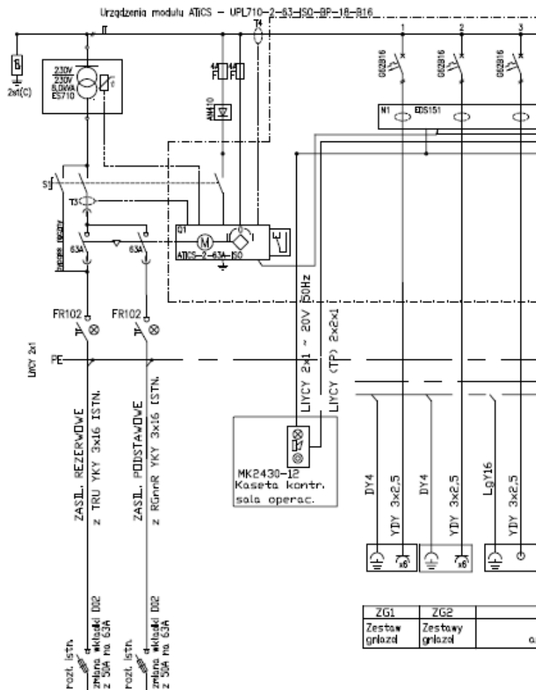
Rys 2a Zasilanie transformatora medycznego/separacyjnego
